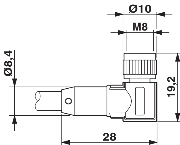
Maßzeichnung
