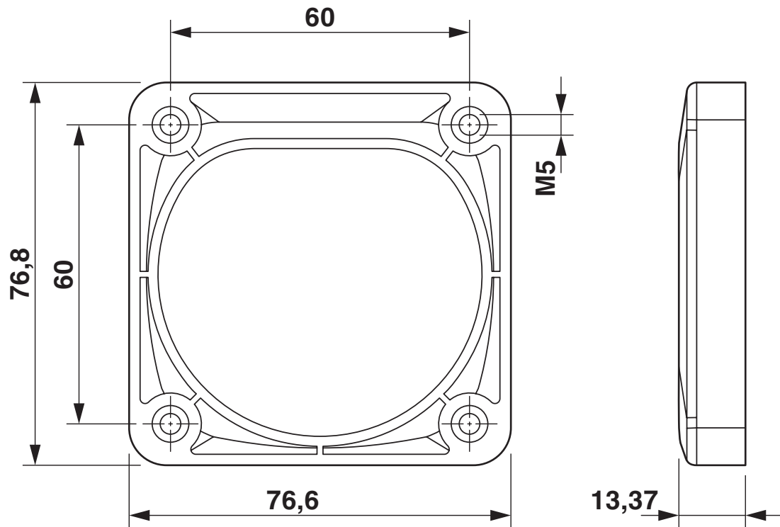
Maßzeichnung
