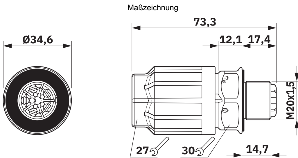
Maßzeichnung des QPD W 5x2,5 M20
