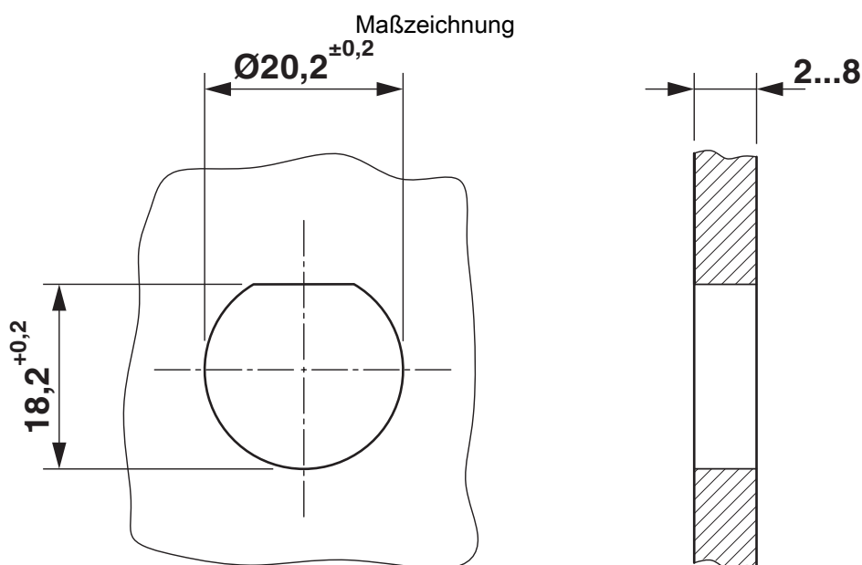
Maßzeichnung des QPD W 5x2,5 M20
