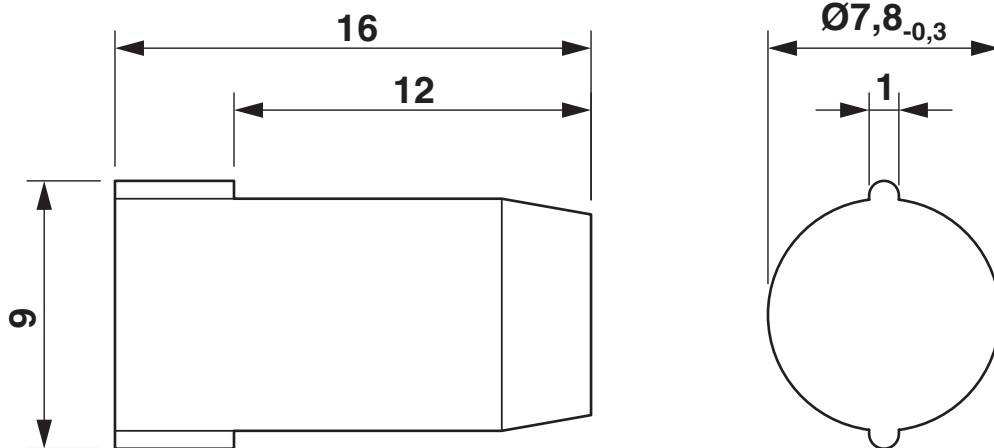
Maßzeichnung
