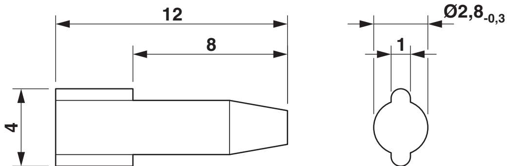
Maßzeichnung
