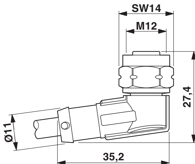
Maßzeichnung
