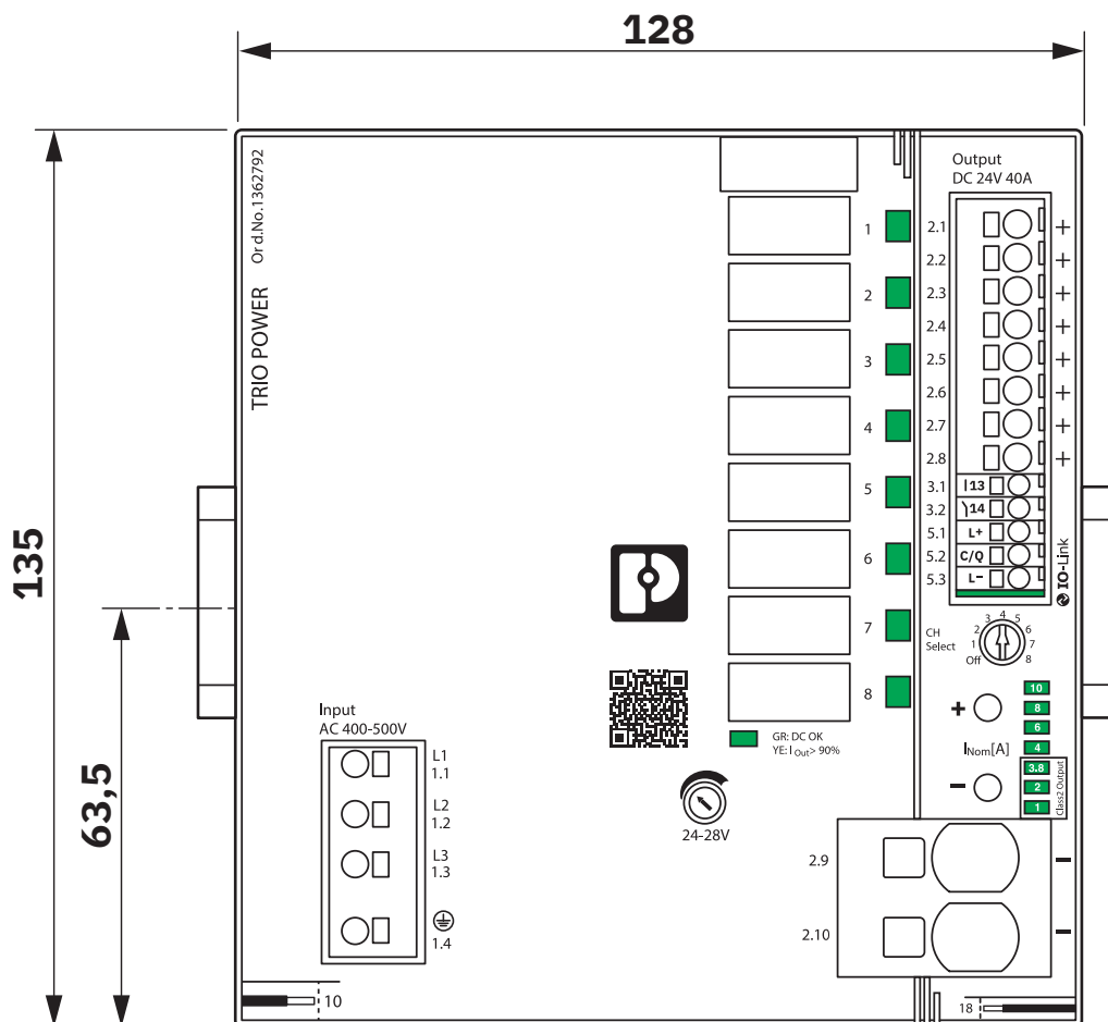
Maßzeichnung
