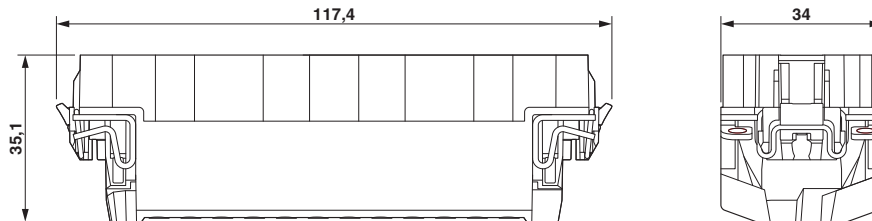
Maßzeichnung
