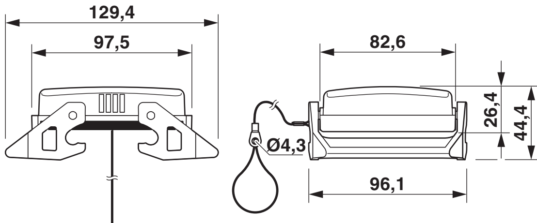
Maßzeichnung
