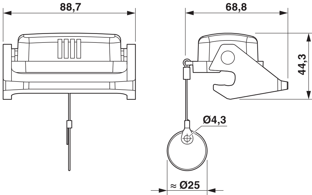
Maßzeichnung
