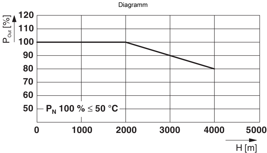
Ausgangsleistung/Aufstellhöhe
