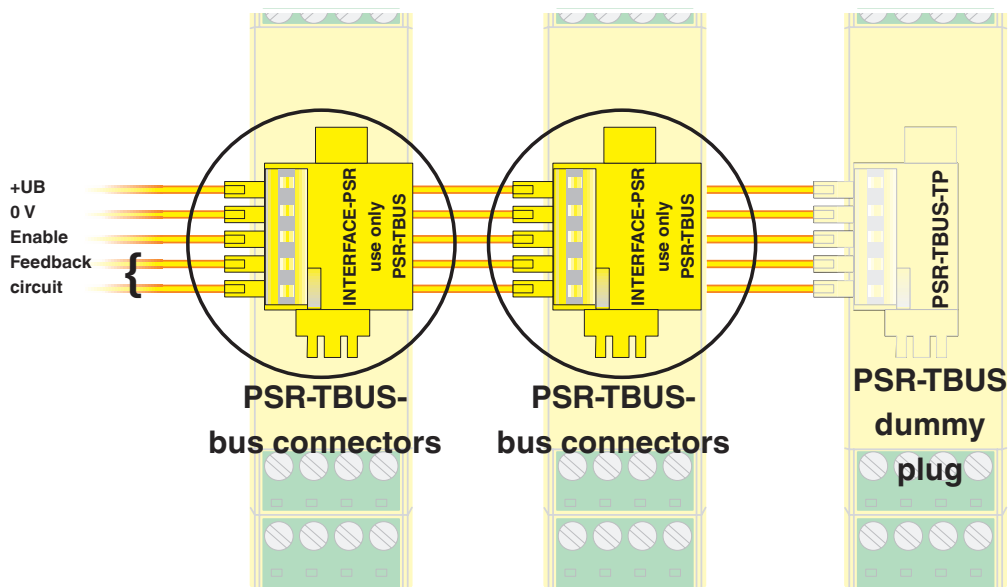
Anschlusszeichnung
