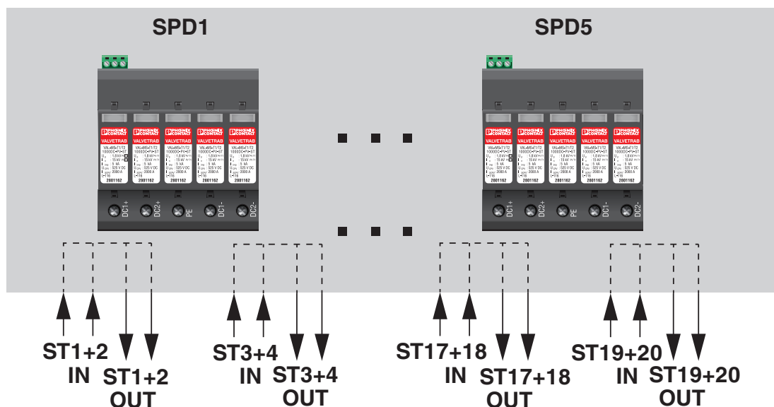
Schematische Applikationszeichnung
