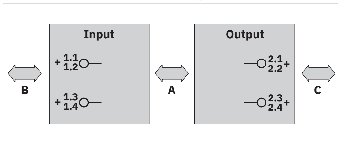
Prüfstrecken Isolationsspannung
