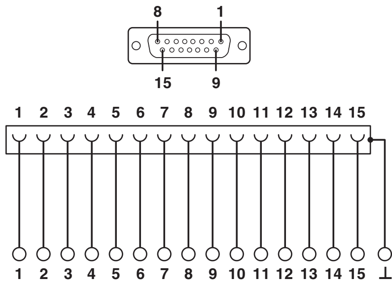
Schaltplan
