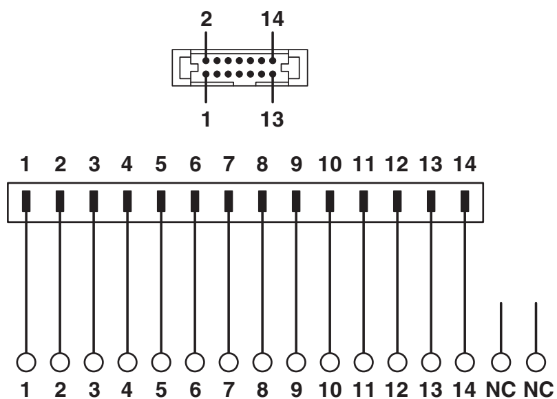
Schaltplan
