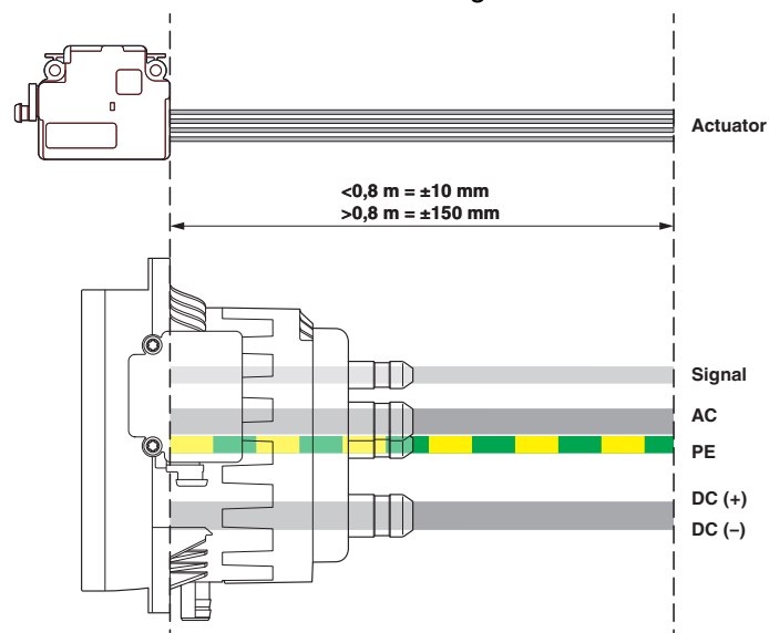
Maßzeichnung
