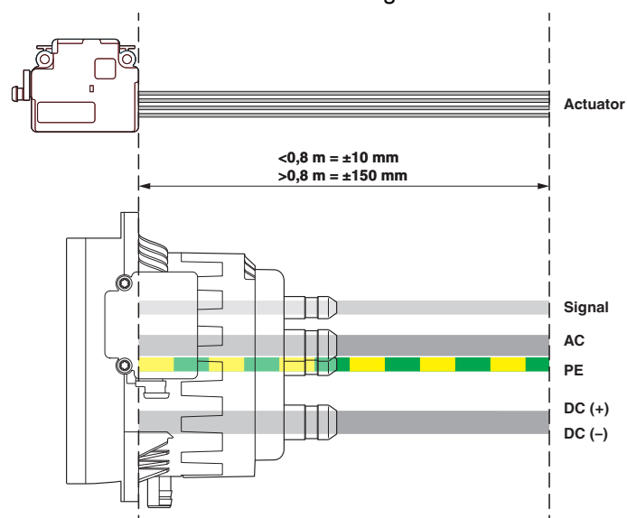
Maßzeichnung
