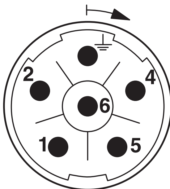
Schemazeichnung
