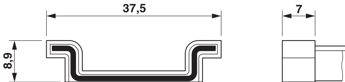
Maßzeichnung
