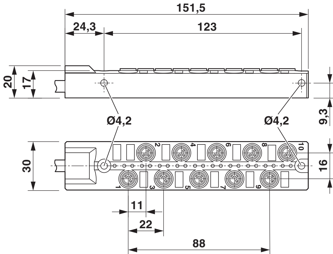
Maßzeichnung
