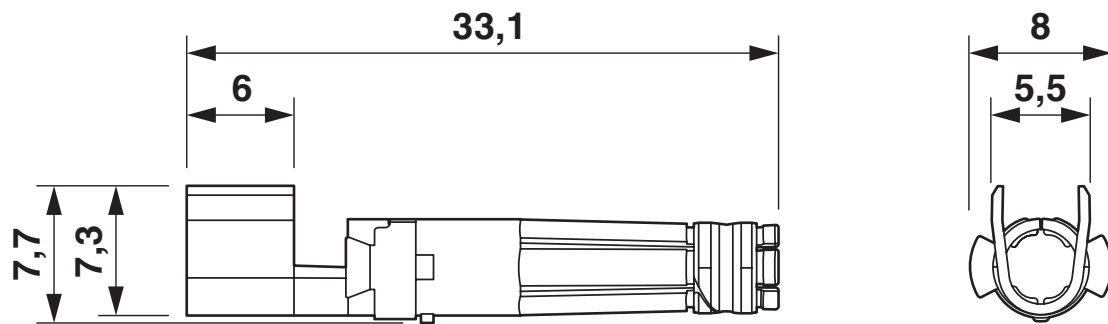
Maßzeichnung
