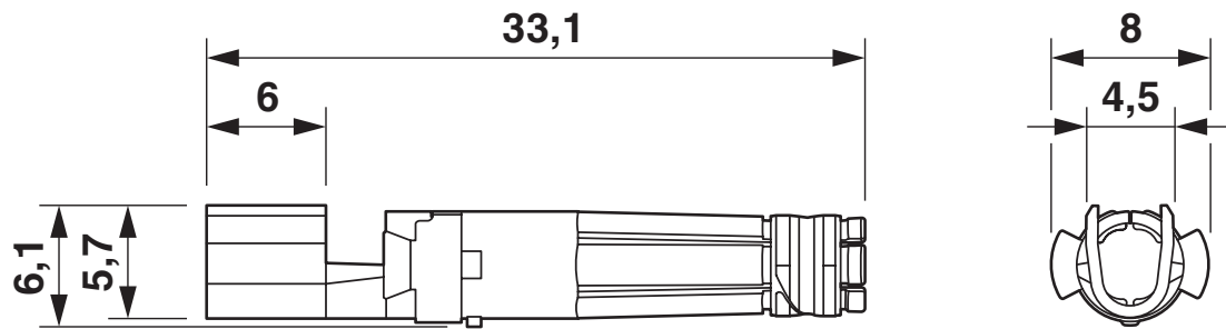
Maßzeichnung
