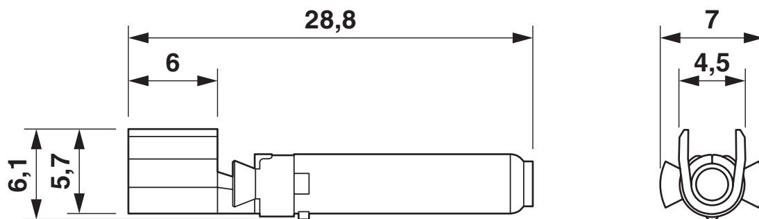
Maßzeichnung
