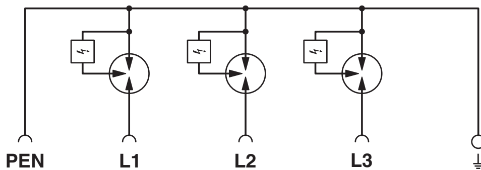
Schaltplan
