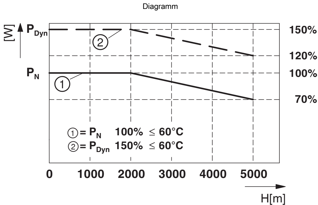
Höhenabhängiges Derating
