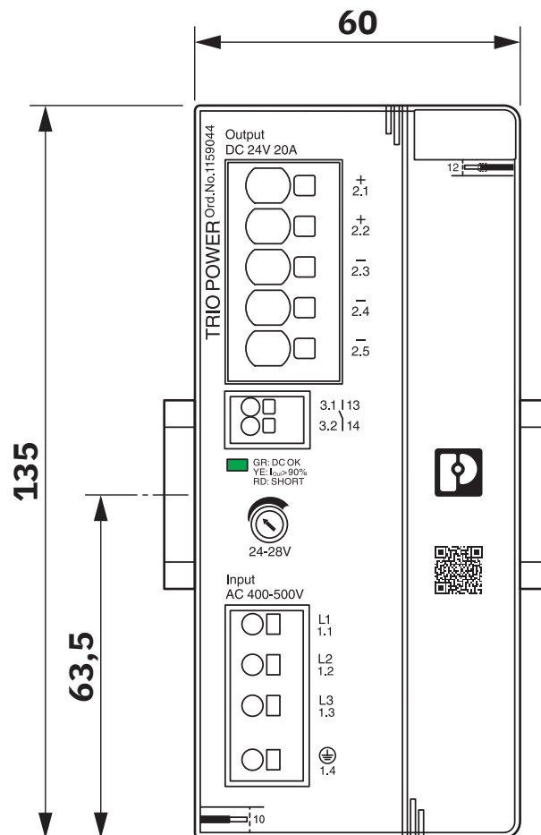
Maßzeichnung
