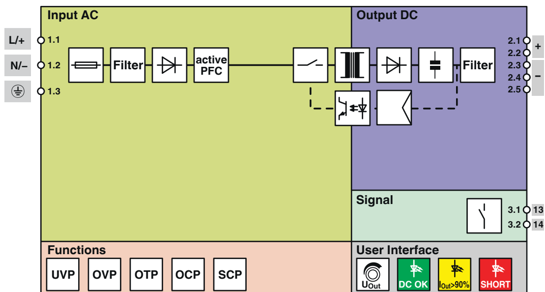
Blockschaltbild
