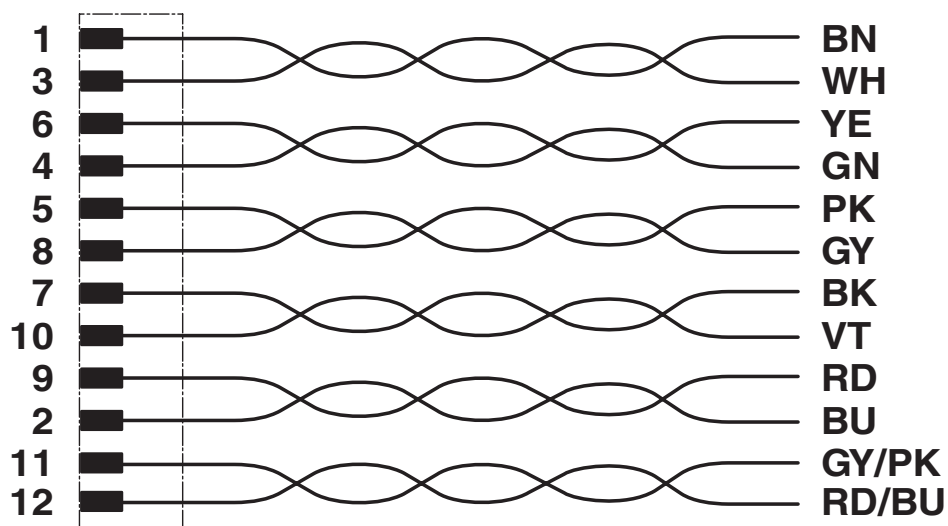
Schaltplan
