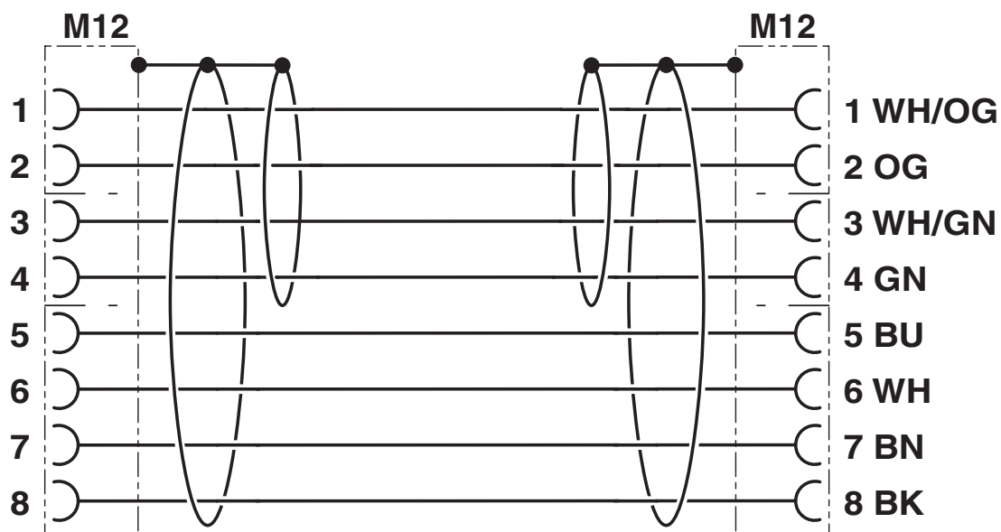
Kontaktbelegung der M12-Buchsen
