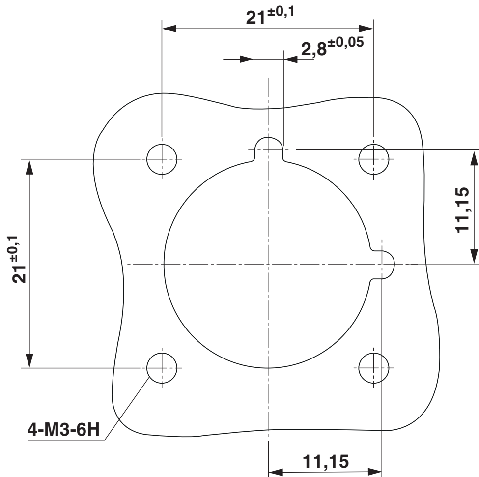
Bohrplan/Lötpadgeometrie
