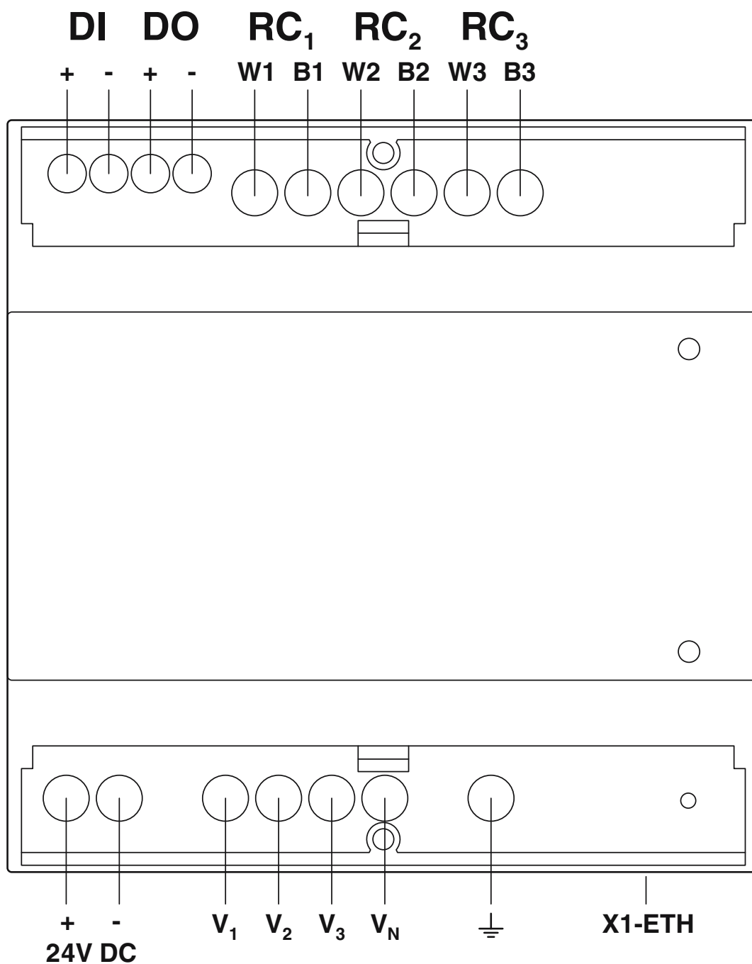
Anschlusszeichnung
