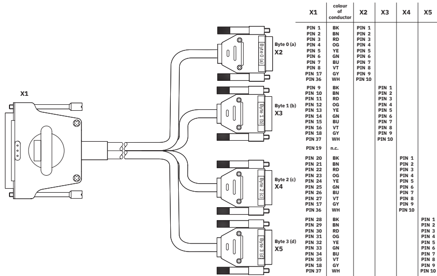
Schaltplan
