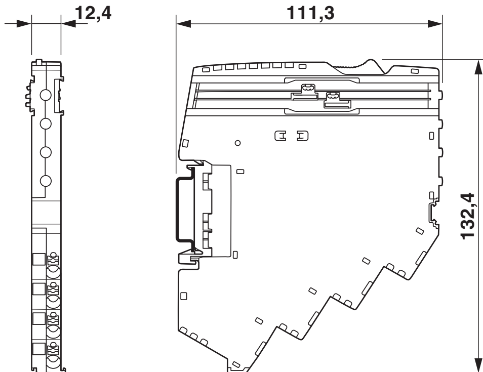
Maßzeichnung
