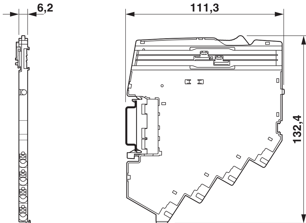
Maßzeichnung
