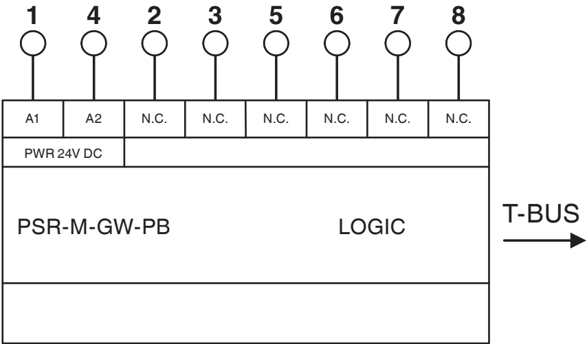
Blockschaltbild
