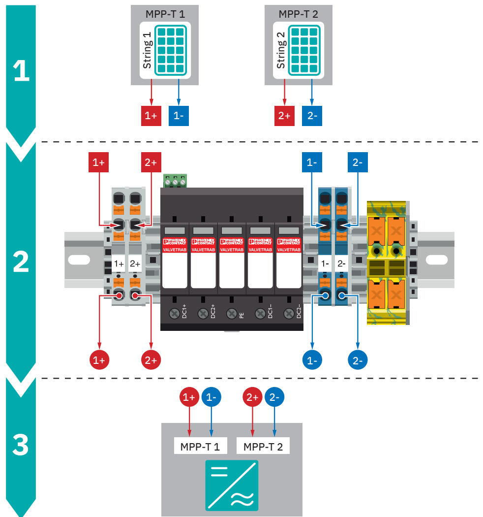
Schematische Applikationszeichnung
