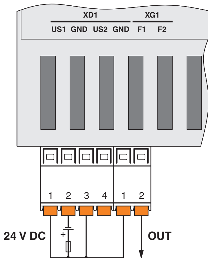
Anschlusszeichnung
