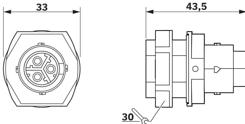
Maßzeichnung
