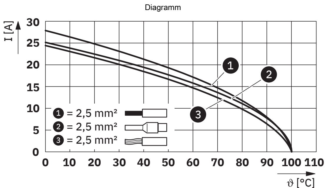
Derating-Diagramm für 2,5 mm²
