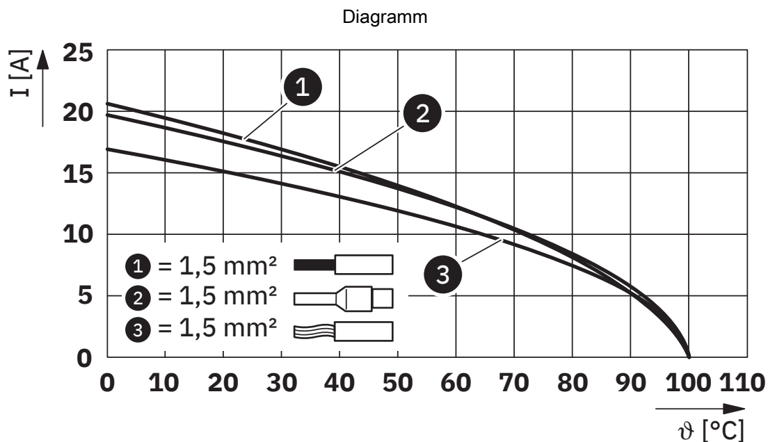
Derating-Diagramm für 1,5 mm²
