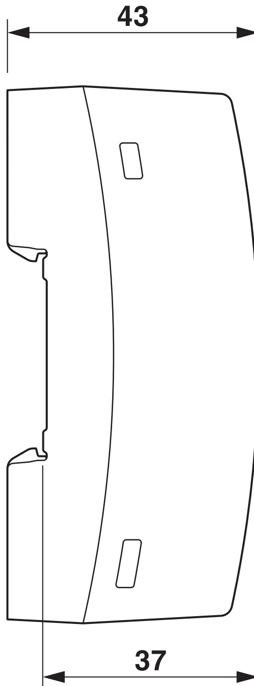
Maßzeichnung
