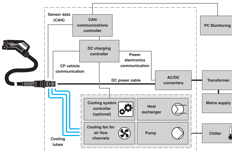
Schemazeichnung
