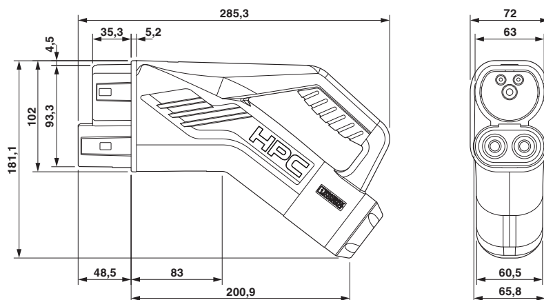
Maßzeichnung
