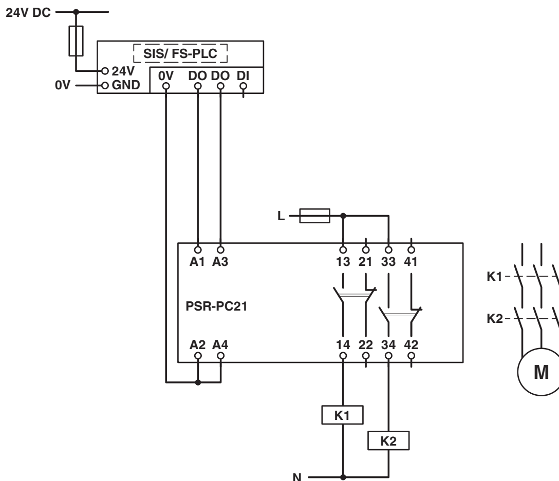
Schaltplan
