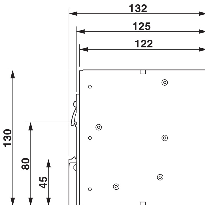
Maßzeichnung
