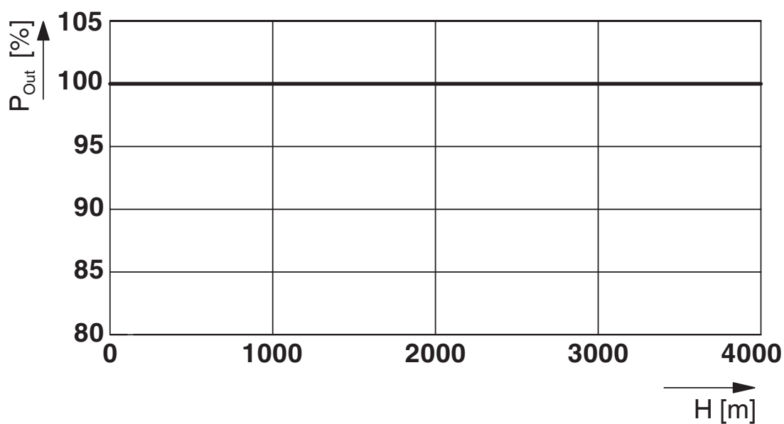
Ausgangsleistung/Aufstellhöhe
