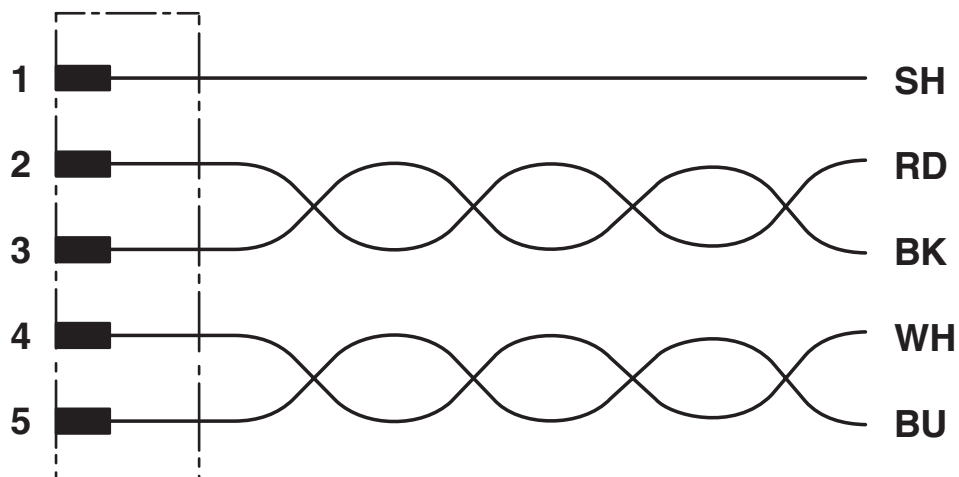
Schaltplan
