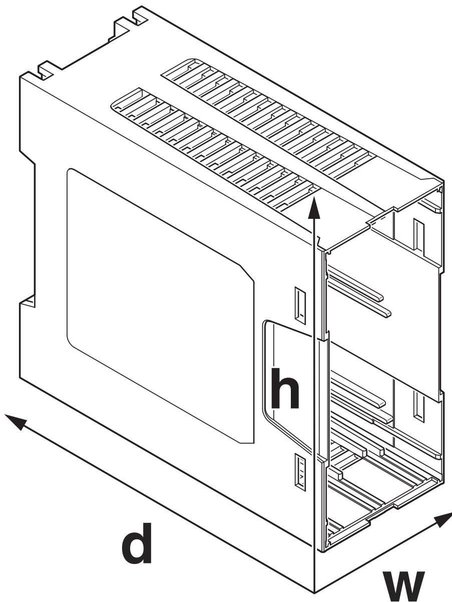
Maßzeichnung
