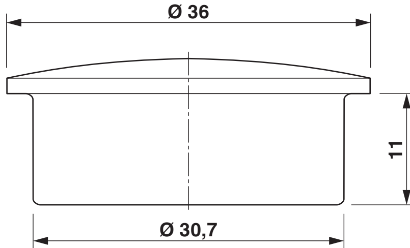
Maßzeichnung
