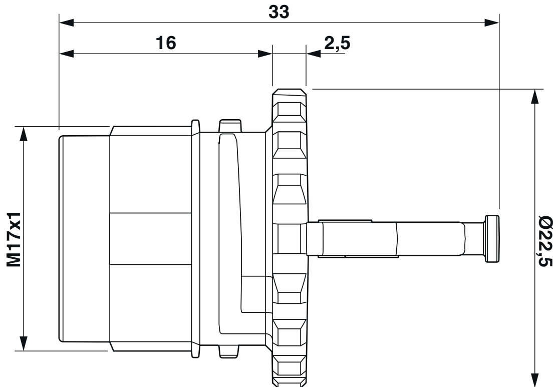
Maßzeichnung
