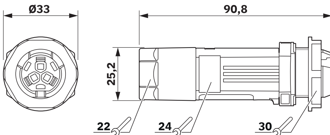
Maßzeichnung
