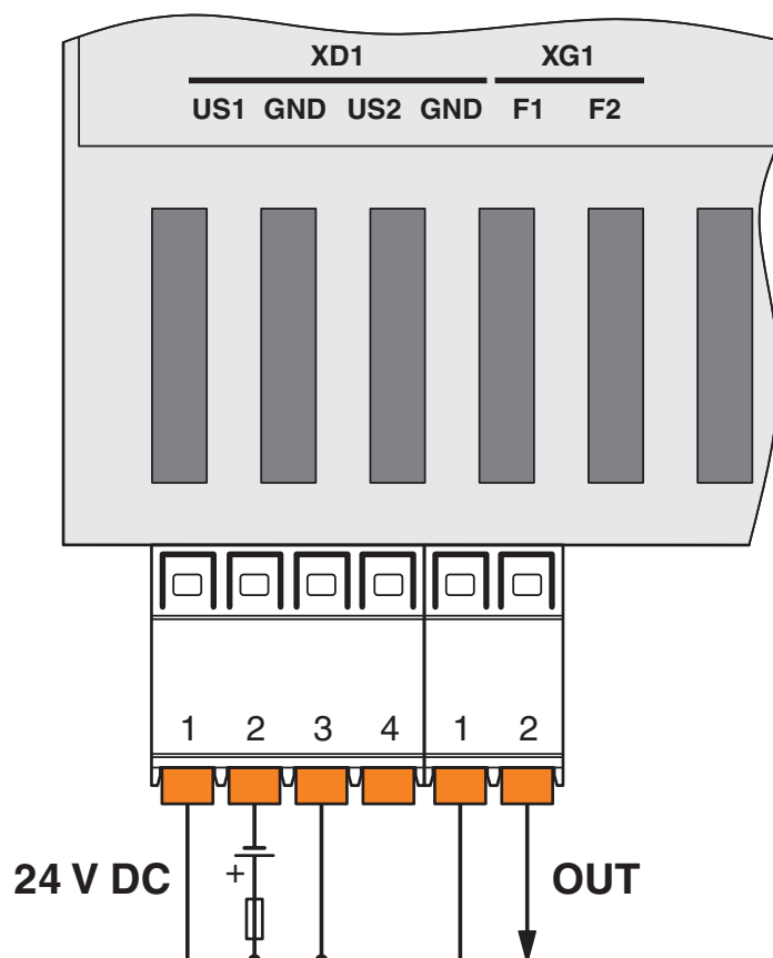
Anschlusszeichnung
