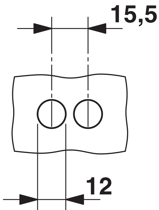
Maßzeichnung
