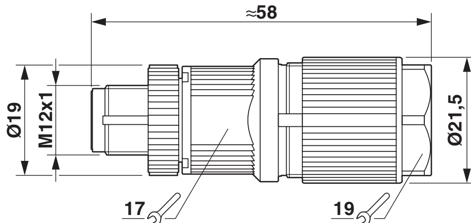
Maßzeichnung
